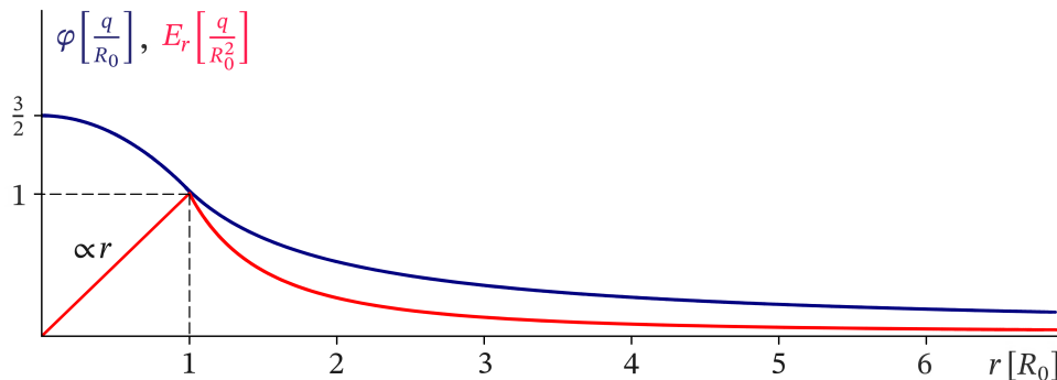
Abb. 1.2-1: Die Graphen der Funktionen \varphi(r) und E_r(r)
