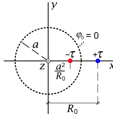
Ersatzproblem für R > R_0
