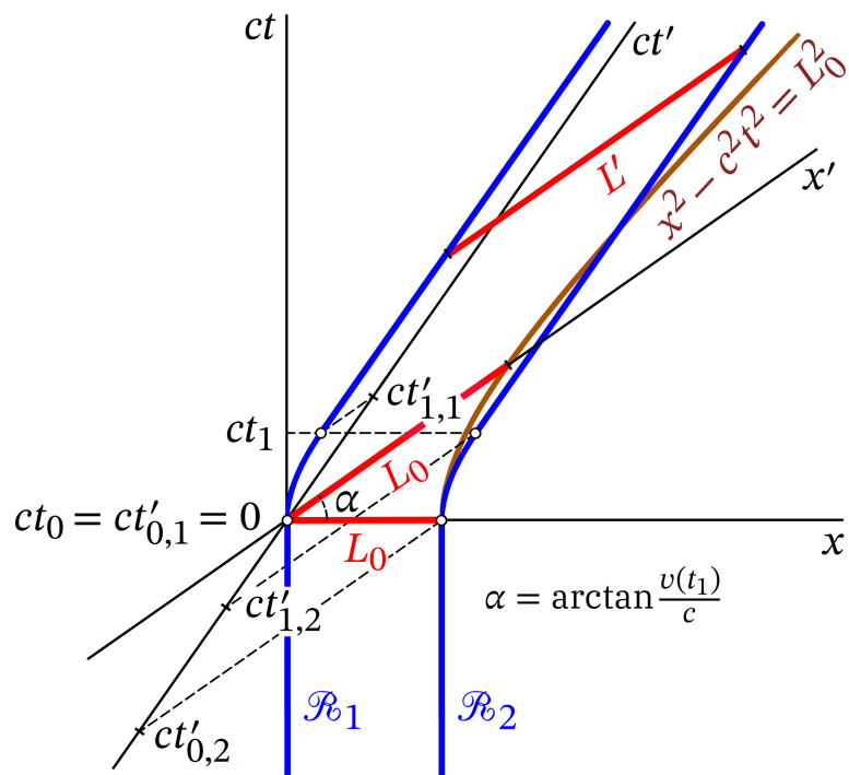
Abb. 9.11 -1: Für die Zeichnung wurde \gamma(v(t_1)) größer gewählt als im Zahlenbeispiel der Aufgabe, damit der Effekt deutlich sichtbar ist; in der Aufgabe \gamma = 1,02 ( \alpha = 10,9^\circ ), in der Abbildung \gamma = 1,4 ( \alpha = 35^\circ ).
