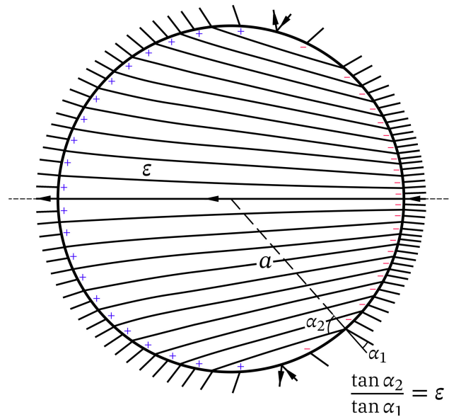
Abb. 3.4-1: Feldlinienverlauf des \mathbf{E} -Feldes in der Umgebung der Kugeloberfläche und im Kugelinneren für den Fall \varepsilon = 2 und r_0 = 3a (Rotationssymmetrie bzgl. der z -Achse; Zeichnung für q > 0 )
